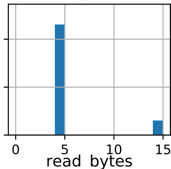
md_mod
