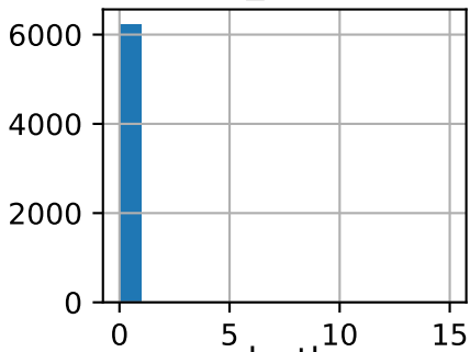
md_other
